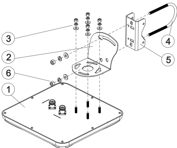
Рисунок 2 - Сборка антенны
